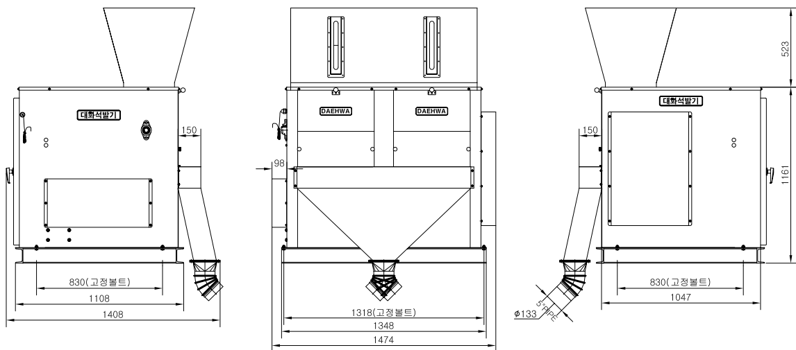
석발기 외형도, 돌식Ⅱ (더블) 7t/h 현, 백미용
