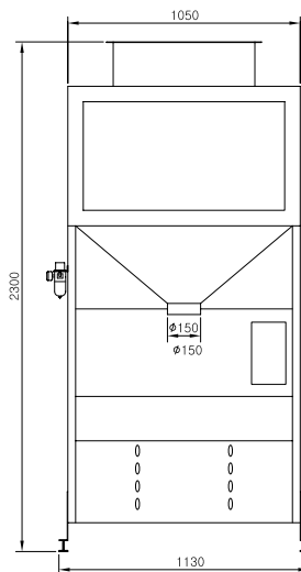
2연식 자동계량기(DP-2) (계량범위 20kg)
