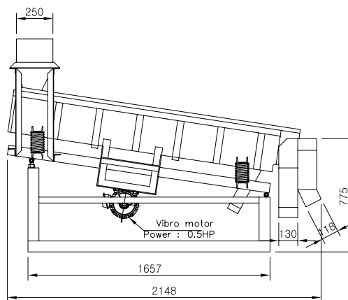
진동선별기 외형도 3.5t/h 청치, 싸라기용
