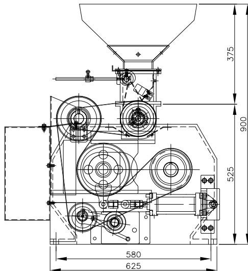
현미기(MJH-SBCA) 3~3.5t/h
