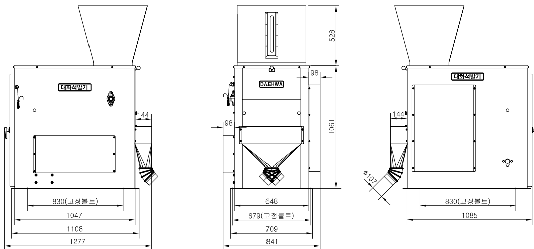
석발기 외형도, 돌식II (싱글) 3.5t/h 현, 백미용
