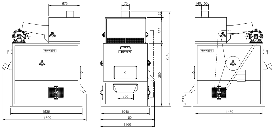
석발기 외형도, 돌쇠(45B) 3t/h 벌 석발용
