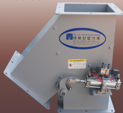
자동 투웨이 게이트
