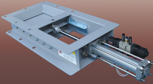
자동 슬라이드 게이트
