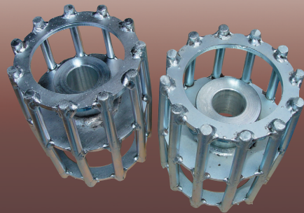
승강기하부드럼(주문사양)
