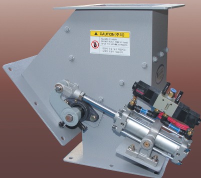
자동 투웨이 게이트
