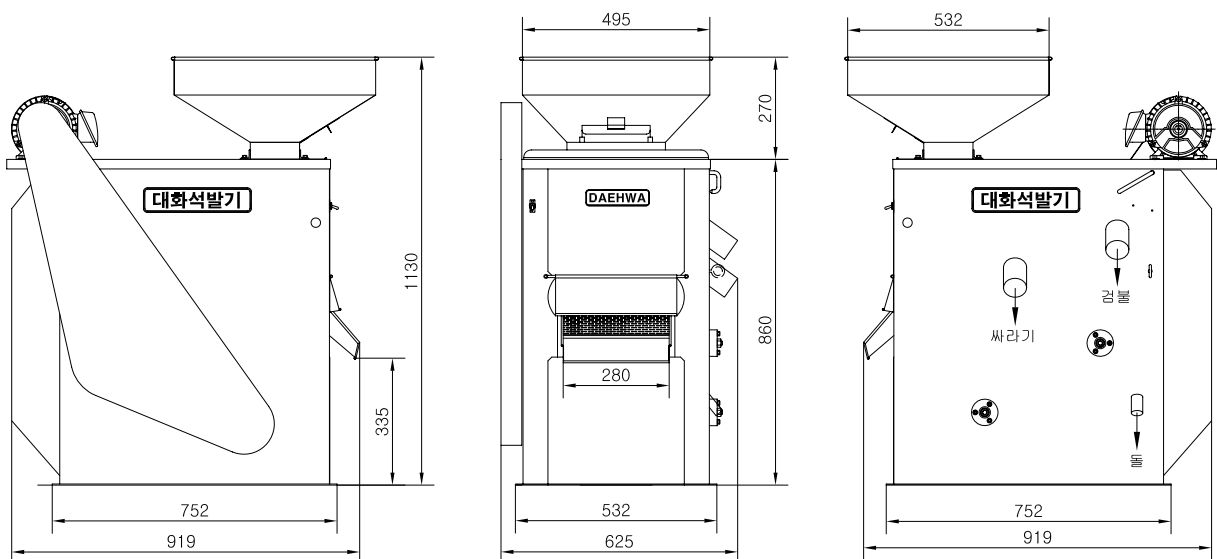
석발기 외형도, 돌쇠(다목적용) 0.6t/h 현, 백미용
