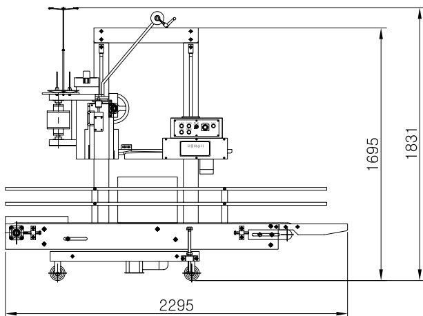
자동미싱기 SJ-50A-1
