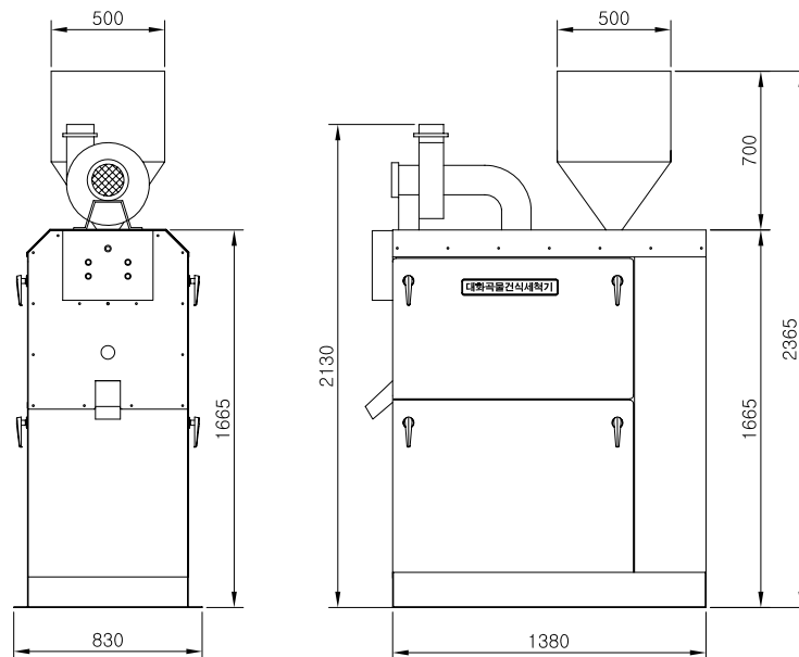
곡물건식세척기(DDP-3)
