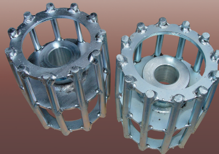
승강기하부드럼(주문사양)
