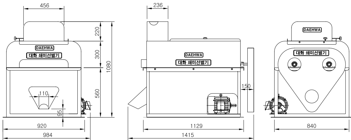
쇄미선별기 외형도(중형) 3t/h 청치, 싸라기용
