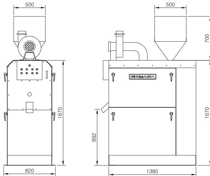
곡물습식세척기(DWP-3) 두태(豆太) 전용
