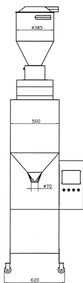
1연식 소포장기+진공이송기(DPS-1) (계량범위 5kg)
