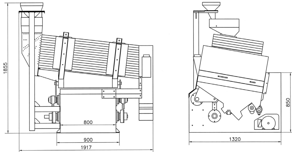
현미분리기 외형도
