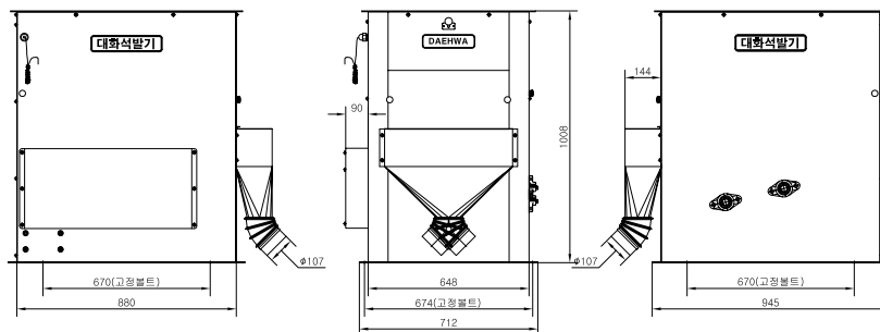
석발기 외형도, 돌쇠(싱글) 3.5t/h 현, 백미용
