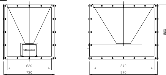
석발기 외형도, 돌쇠(싱글) 3.5t/h 현, 백미용
