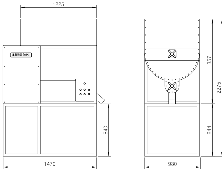
곡물혼합기(DM-2)
