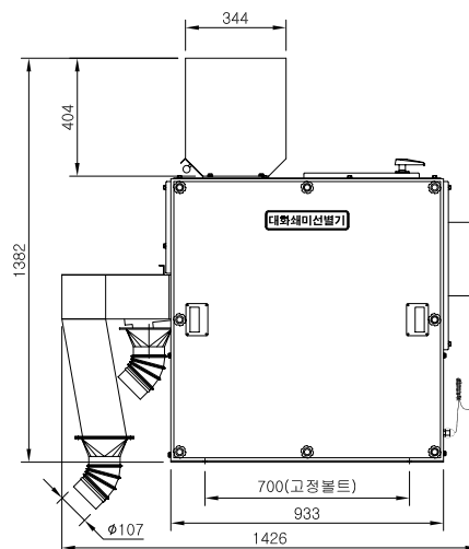
쇄미선별기 외형도 3.5t/h 청치, 싸라기용
