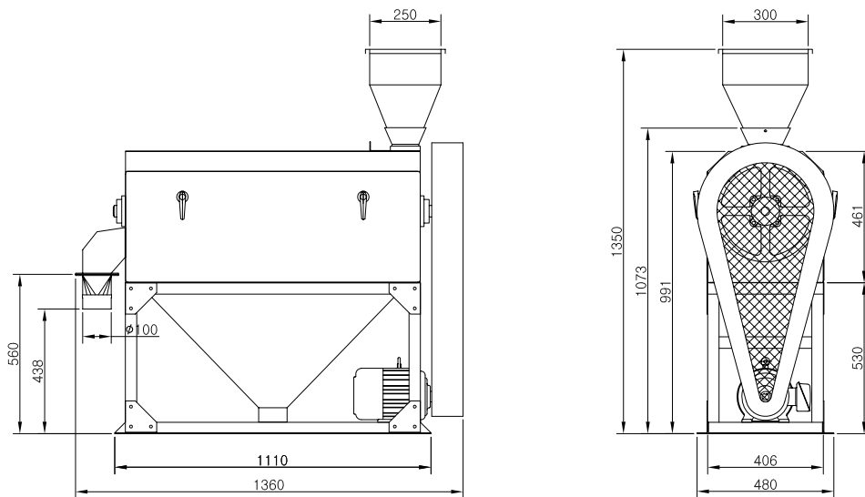
제강기 외형도 3t/h 청치, 싸라기용
