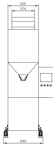
1연식 소포장기(DPS-1) (계량범위 5kg)
