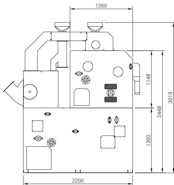
종합석발기(ISPC-60) 6~7t/h 버 석발용
