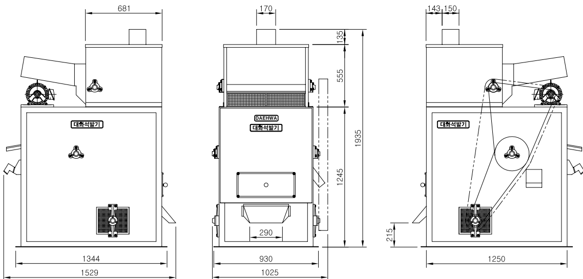
석발기 외형도, 돌쇠(40B) 2t/h 베틀 석발용
