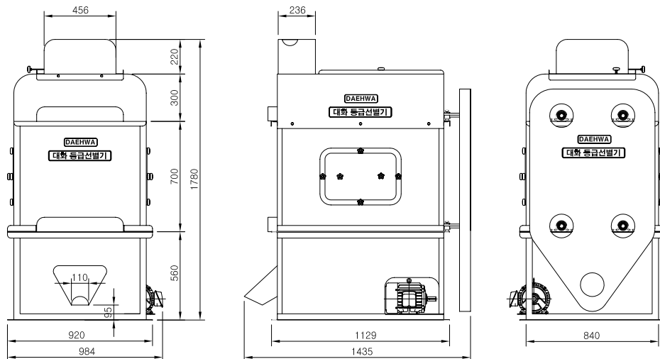
등급선별기 외형도 2t/h 청치, 싸라기용
