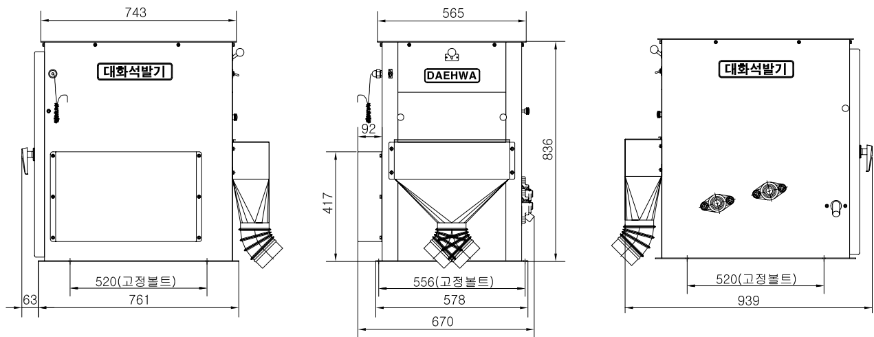
석발기 외형도, 돌쇠(소형) 2t/h 현, 백미용
