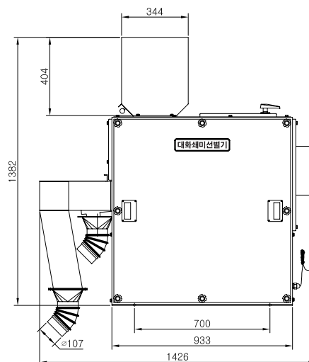
Broken Rice Separator(Swaedori)
