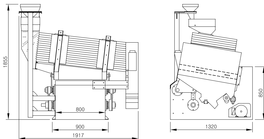
Paddy Separator (ISPS-35)
