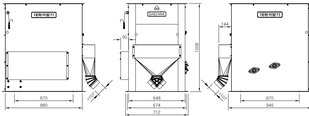
Stone Separator Dolsoe
